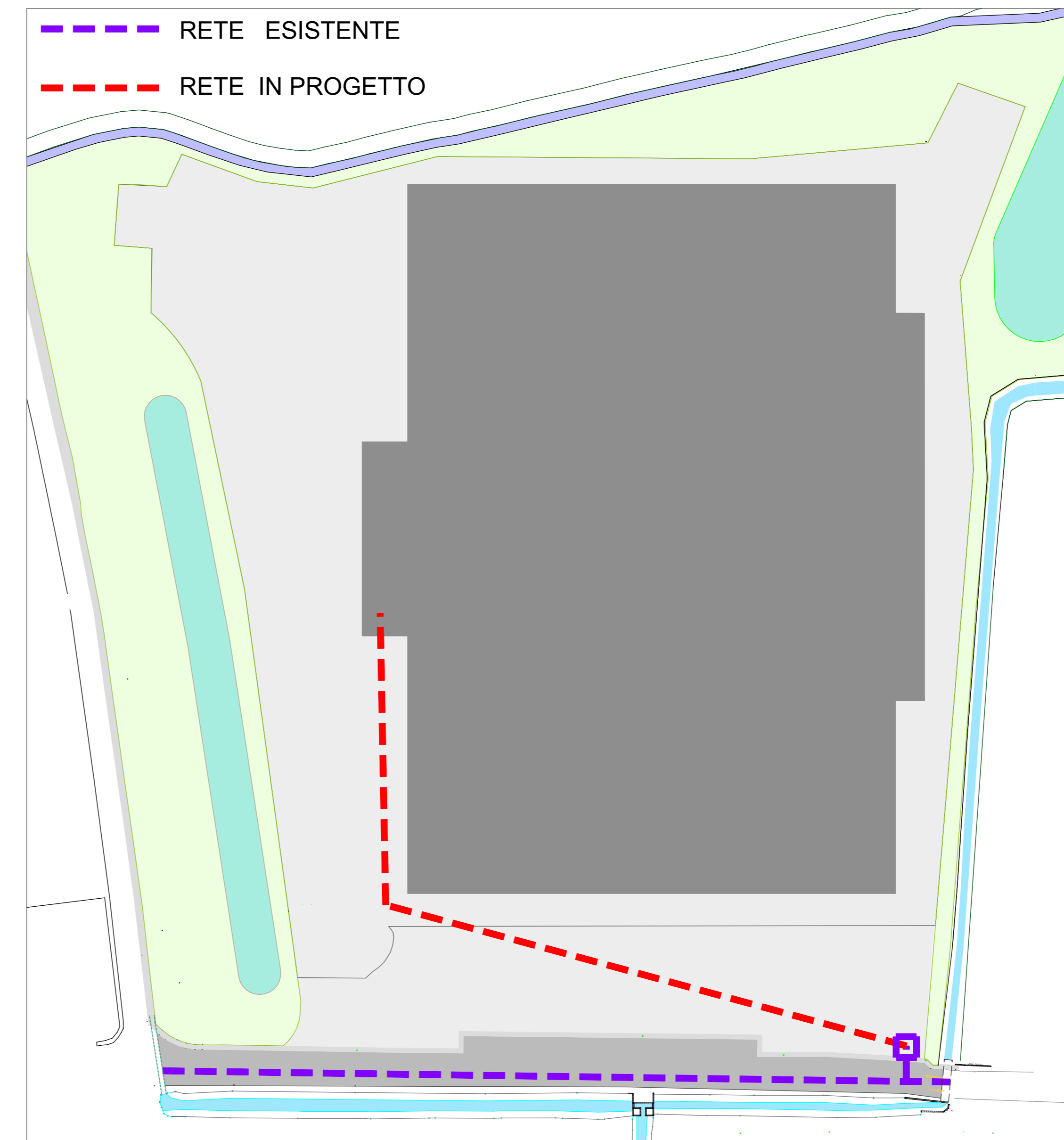
RETE ACQUEDOTTO
