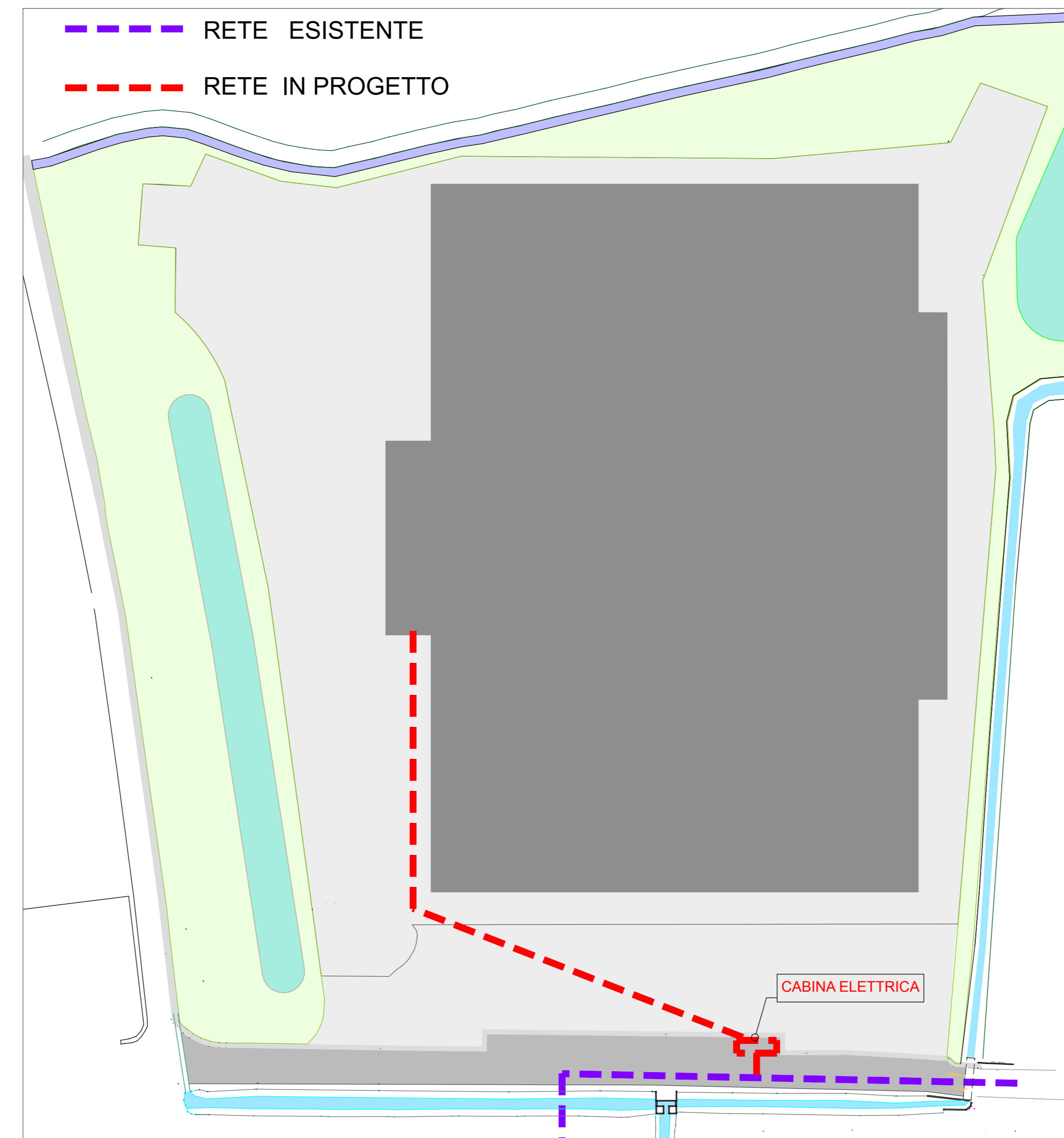
RETE LINEA ELETTRICA
