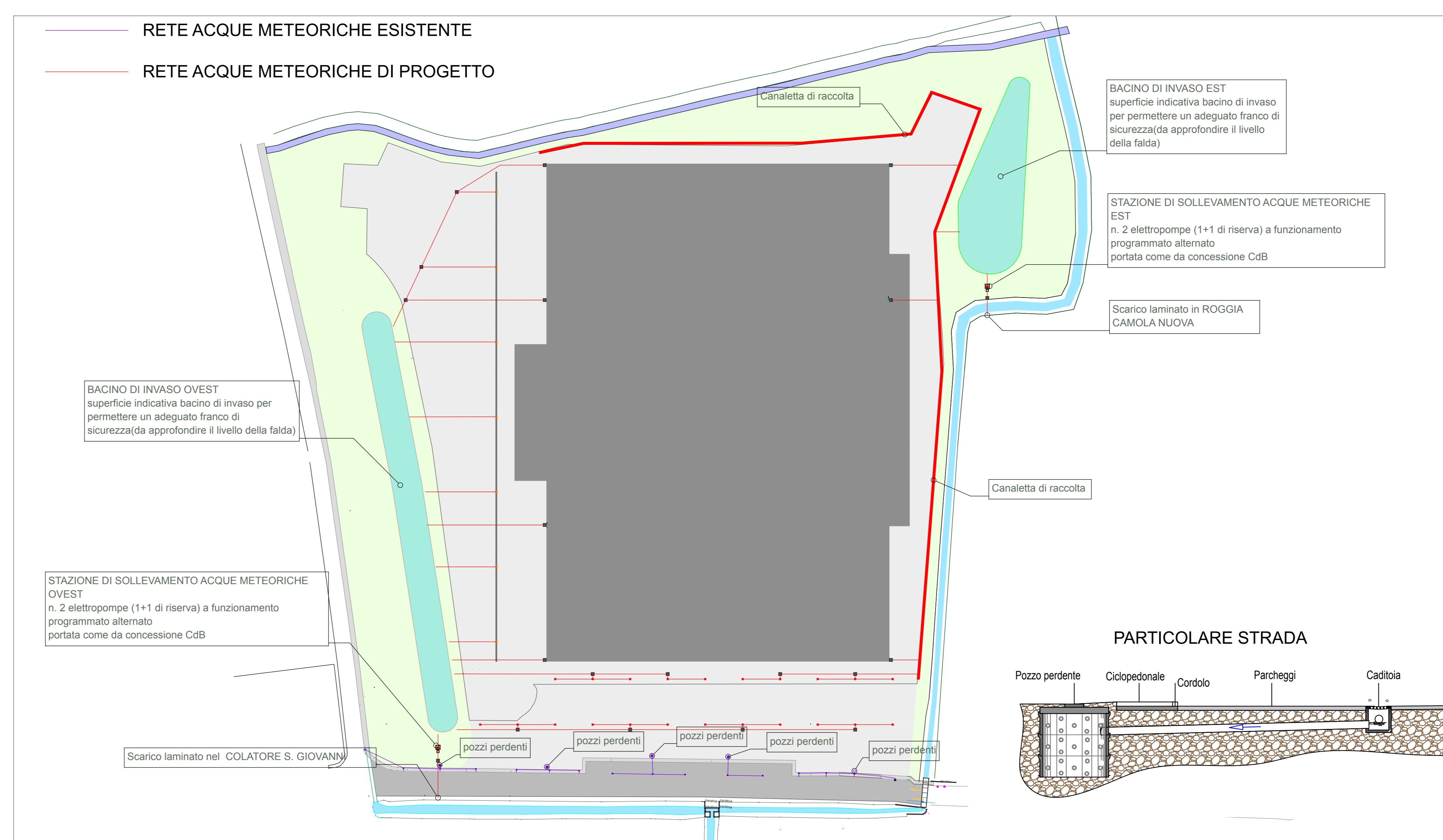
RETE ACQUE METEORICHE
